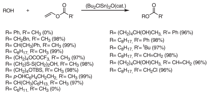
Scheme 1-86
