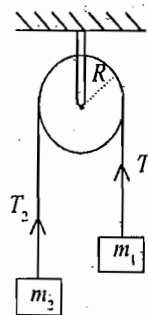
Fig 1.12 : Atwood machine (Pulley having mass M)
