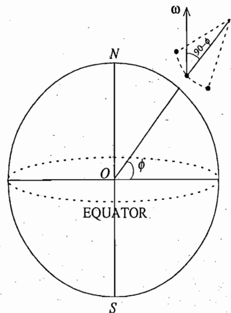
Fig. 11.7 : Foucault's pendulum
