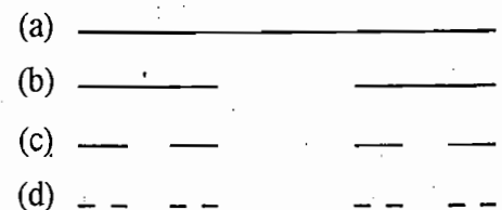
Fig. 16.29. Cantor set
