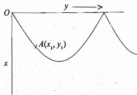
Fig. 5.7 : Cycloid
