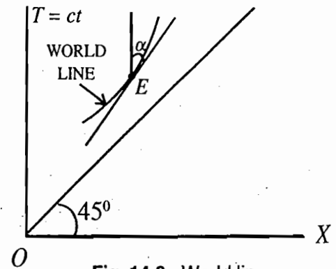
Fig. 14.2 : World line
