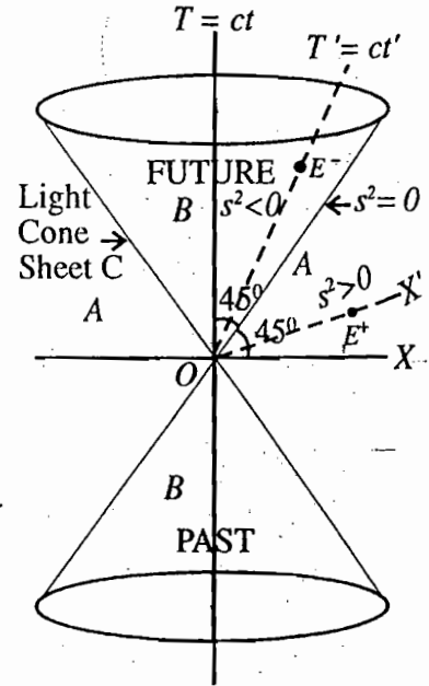
Fig. 14.3 : Light Cones
