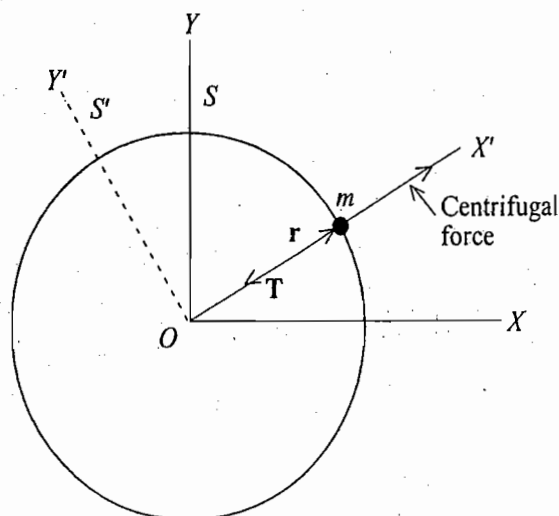
Fig. 11.3 : Centrifugal force
