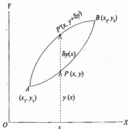
Fig. 5.1 : \delta -variation
