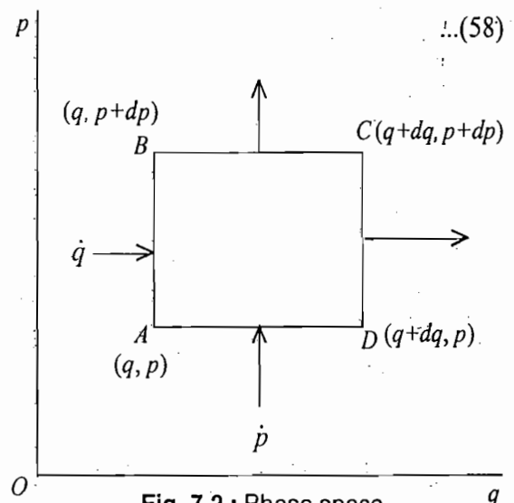
Fig. 7.2 : Phase space
