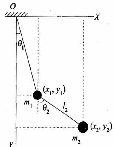
Fig. 9.6 : Double pendulum
